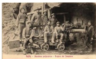
22446. Iselle, Macchina perforatrice, Traforo T2/3 6000
