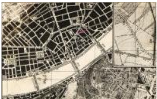
20198. ** Budapest, térkép T2 T2 1400
