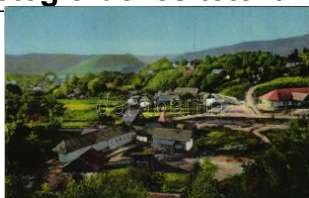
43017. ** Szováta, Sovata; Colonia bailor de j T2 4200
